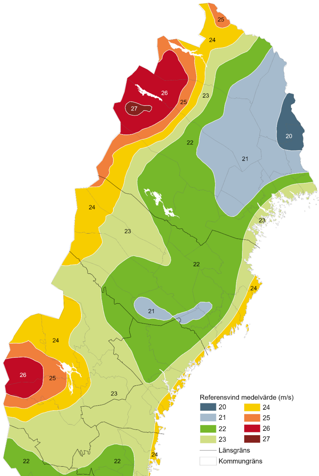
Figur 4:3 Referensvindhastighet, v_b
