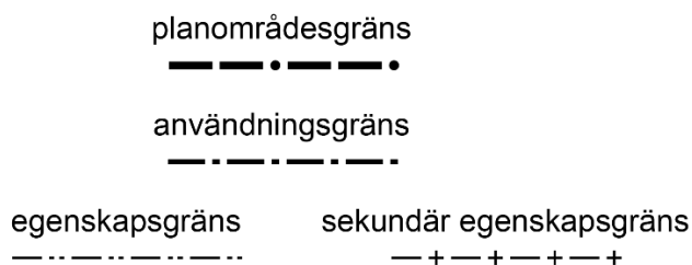
Figur 1: Gränshierarkin
