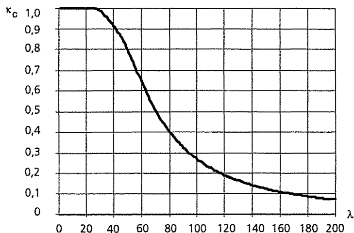
Figur a. Reduktionsfaktorn \kappa_c för konstruktionsvirke med E_{Rk}/f_{ck} = 300 .
