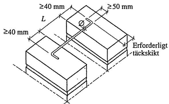
Figur a. Förankring av murkramla.
