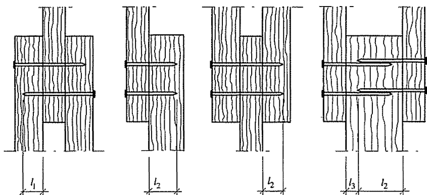
Figur a. Förankringslängd för spik
