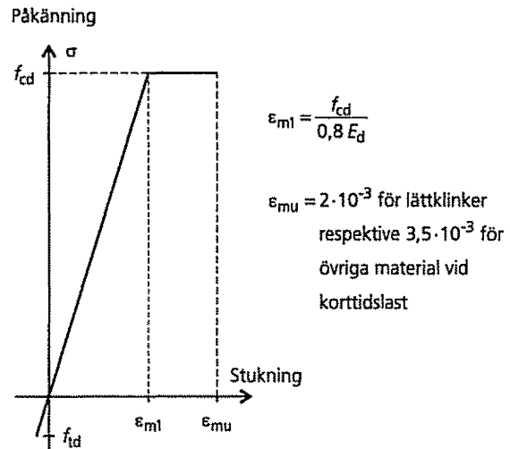
Figur a. Idealiserad arbetskurva för murverk.
