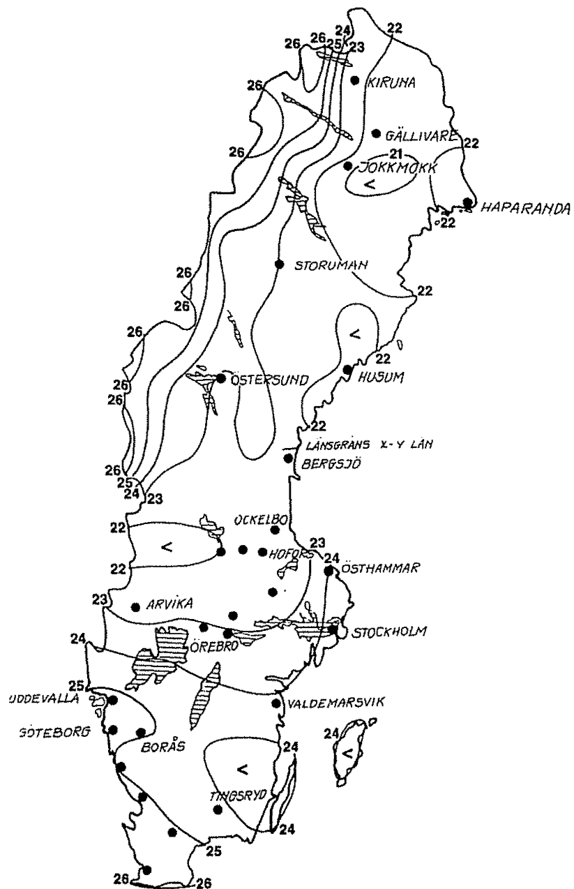
Figur a. Referensvindhastigheten v_{ref} i m/s, dvs. medelvindhastighet under 10 minuter på höjden 10 meter över markyta med råhetsparameter z_0 = 0,05 och med upprepningstiden 50 år.
