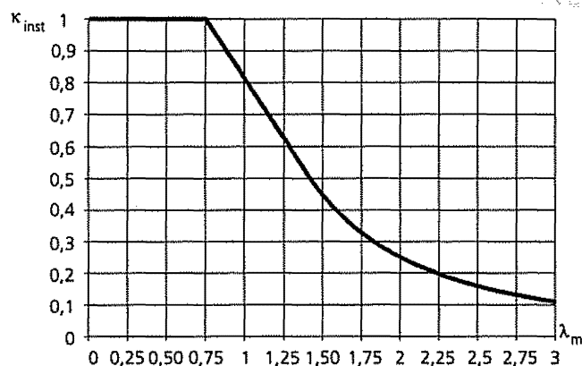
Figur a. Reduktionsfaktorn \kappa_{inst}
